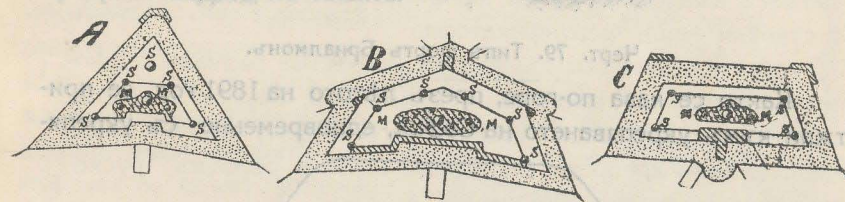
Черт. 78. Схеми на бриалмонови фортове.
