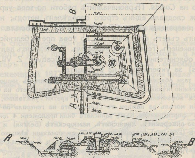
Черт. 79. Типъ фортъ Бриалмонъ.
