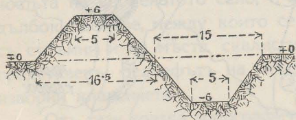
Черт. 11. Профилъ на старобългарски прокопъ—преграденъ валъ.
