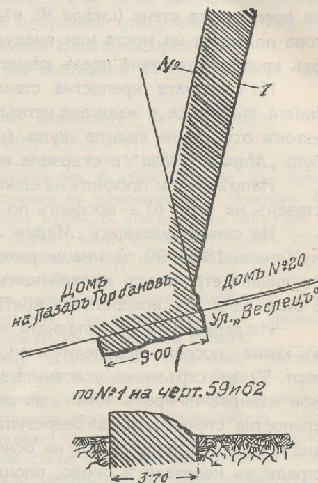
Черт. 62. Остатъци отъ развалини на римска креп. стена на ул. „Веслецъ“.
