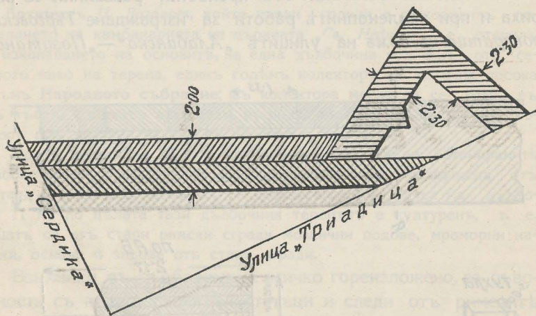
Черт. 64. Развалини отъ основи на вътр. креп. стена — жгълтъ на ул. „Сердика“ — „Триадица“.
