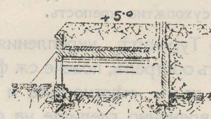
Прорѣзъ по АБ на каземата
