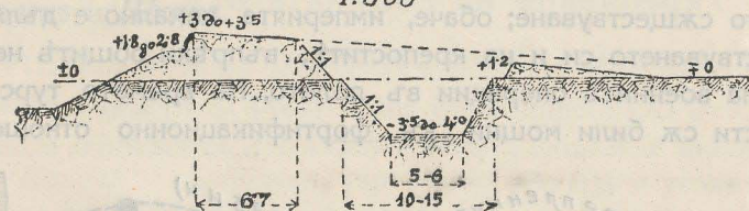
Напрѣченъ разрѣзъ на вrustвe-ра и въ фасадъ-траверсътъ
