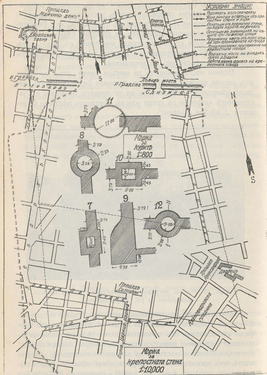
Черт. 59. Планъ на римскитѣ крепостни стени, нанесени върху сегашния планъ на София.
