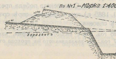
Черт. 76. Планъ на редута „Коньовица“ съ профилъ по №1
