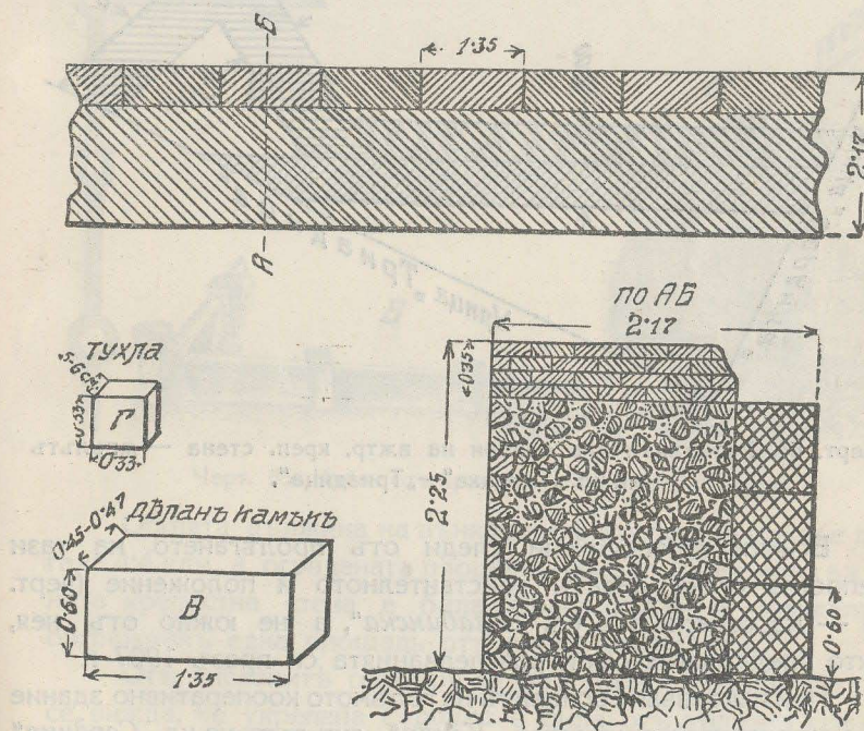
Черт. 63. Развалини отъ южната креп. стена при Сждебната палата.
