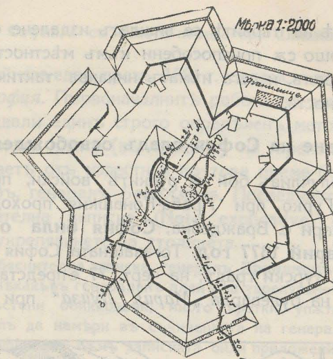
Черт. 75. Планъ на редута „Куру-багларъ“.
