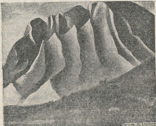
Черт. 8. Часть отъ меловетъ при Мелникъ.
