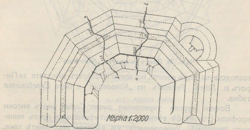
Черт. 73. Планъ на Слатинския лунетъ.
