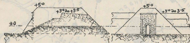
Планъ на траверса
