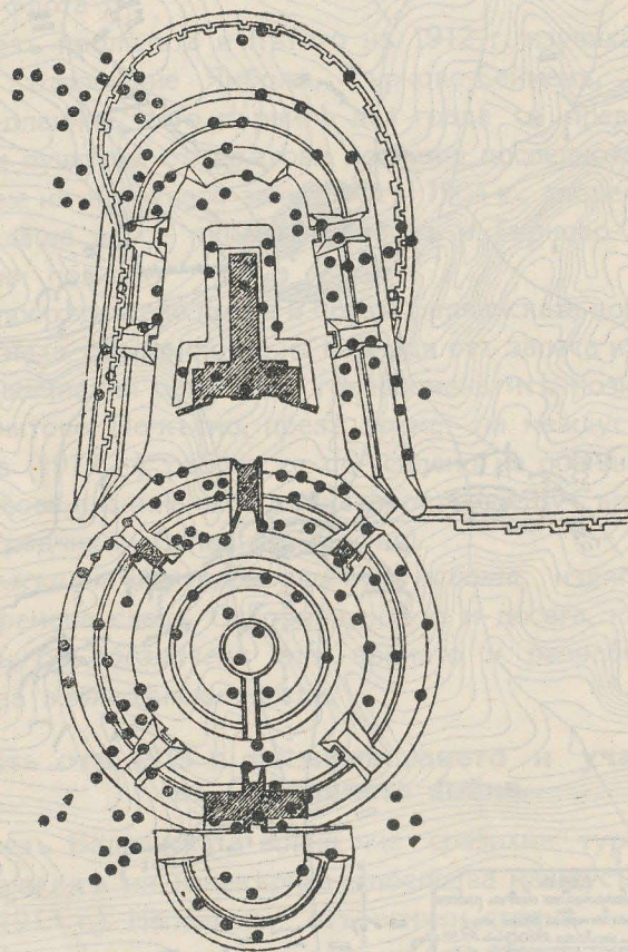
Черт. 92. Фортътъ „Айвазъ-баба“ съ артилерийскитѣ попадения.
