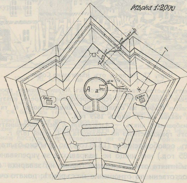
Черт. 75. Планъ на редута „Куру-багларъ“.
