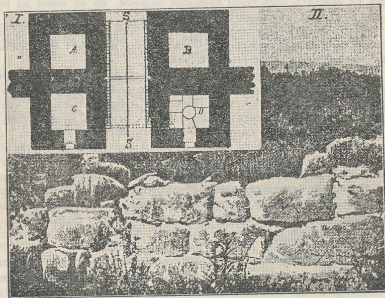
Черт. 36. Планъ на кули и развалини отъ Преславската крепостъ.
