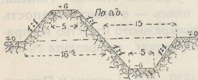
Черт. 13. Профилъ по а б на черт. 12.
