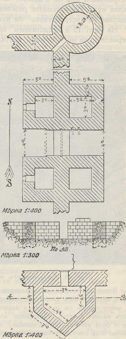
Черт. 14. Планъ на кулитъ по вътрешната ограда.
