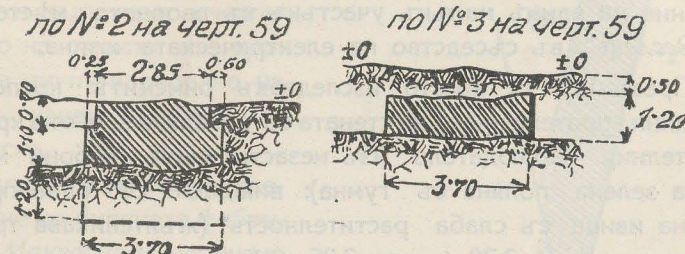
Черт. 60. Профилъ на креп. стена между „Мария-Луиза“ и „Царъ Борисъ“.
