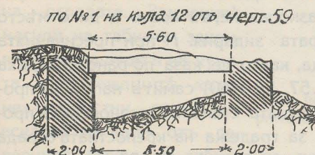
Черт. 61. Профилъ на развалини отъ основитѣ на кръгла кула.
