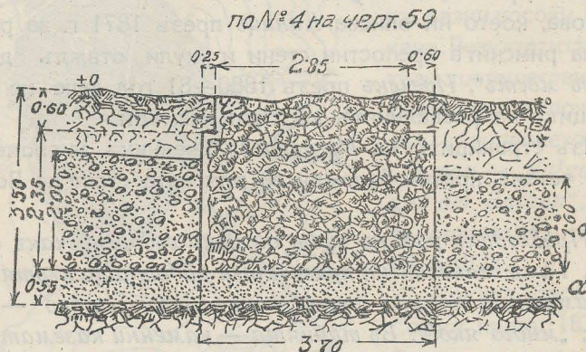
Черт. 57. Профилъ на подтеренни римски креп. развалини на бул. „Хр. Ботевъ“.
