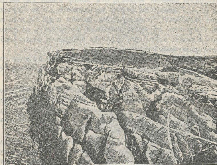
Черт. 26. Перспективенъ изгледъ на крепостнитѣ развалини — „Градътъ“.
