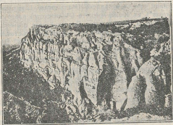
Черт. 23. Мадарскитѣ скали.
