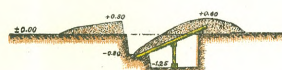
Разрѣзъ по № 2
