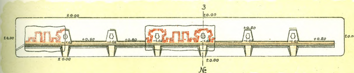
Батарея за 10,5 и 12 см. оръдия.
