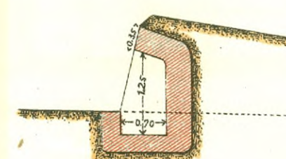
Разрѣзъ по № 5
