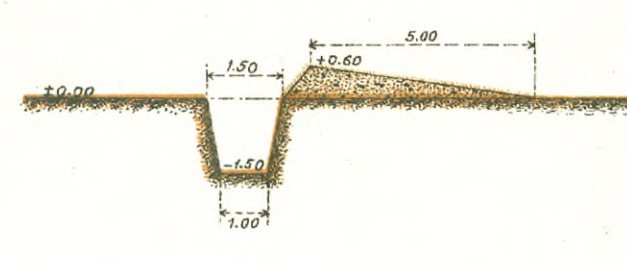
Разрѣзъ по № 3
