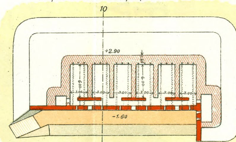
Погребъ (хранилище). — новъ типъ. Мѣрката за плана и разрѣза е 1:400.
