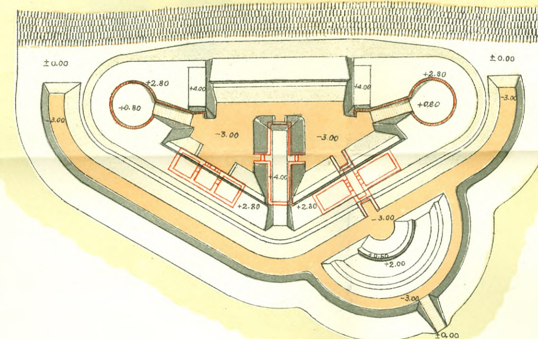
IX Фортъ Ташлъкъ-Алтъ
