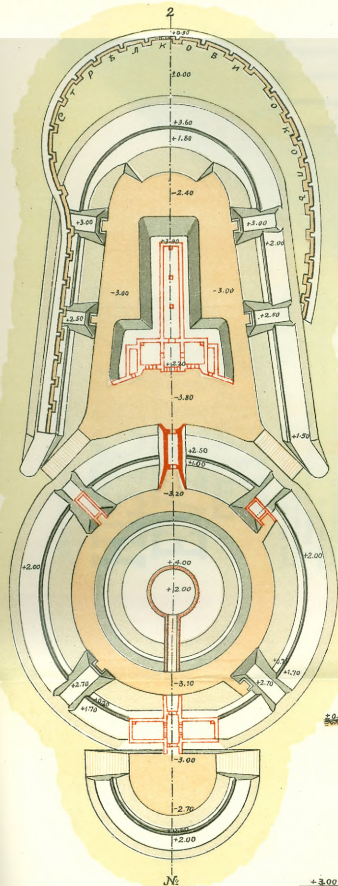
ХІІІ. Фортъ Айвасъ-Баба
