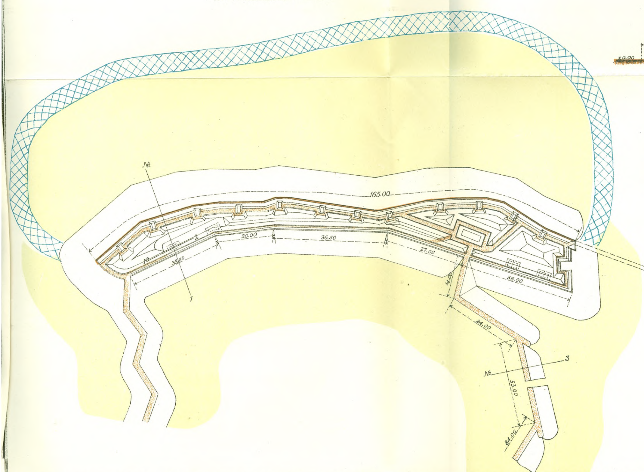
Редута при гробищата. Въ С. Западна секторъ.
