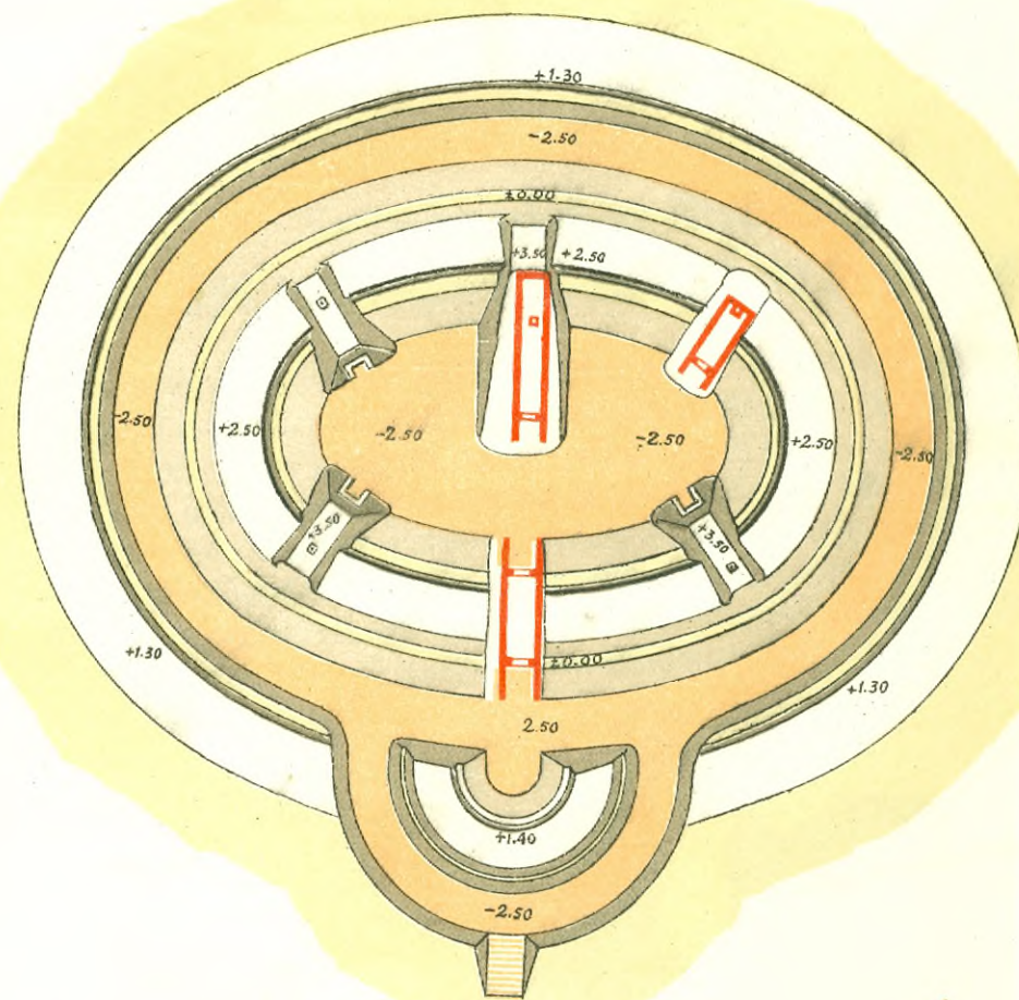
XVI. Фортъ Куру-Чешме
