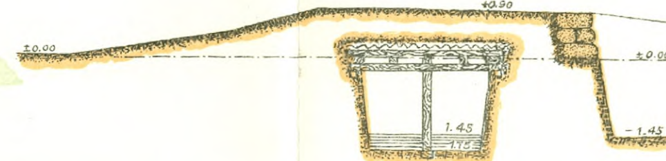
Разрѣзъ по № 2
