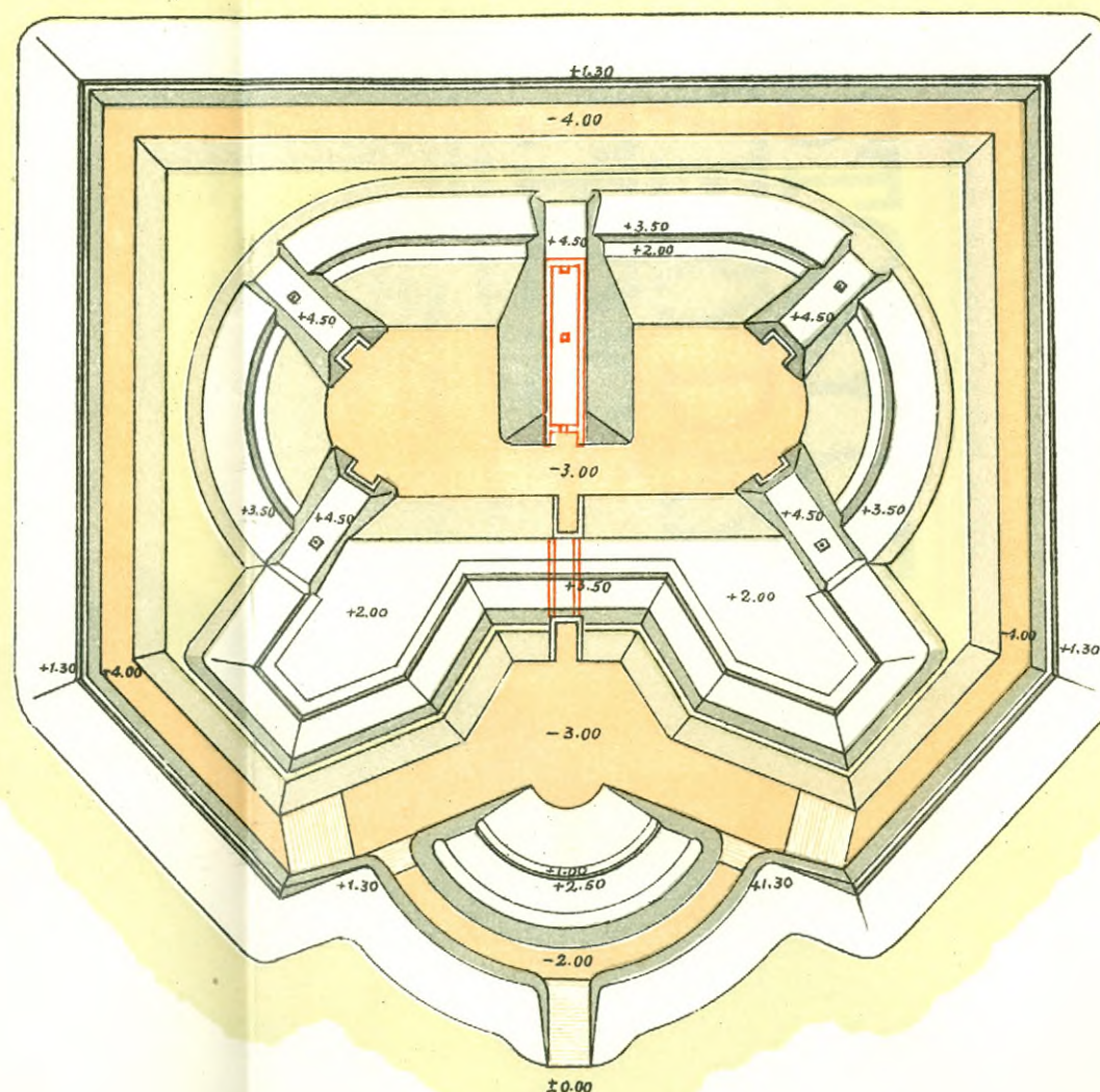
ХХVI. Фортъ Марашъ
