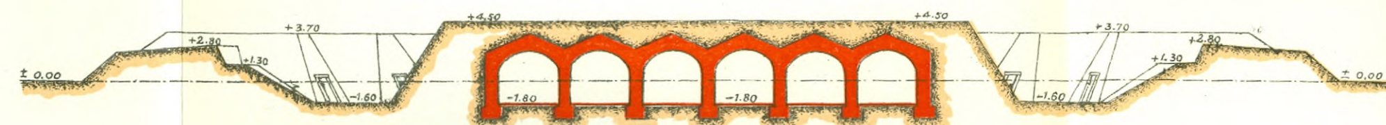
Междина батарея за 10.5, 12 и 15 см. оръдия (безъ бетонни постройки).
