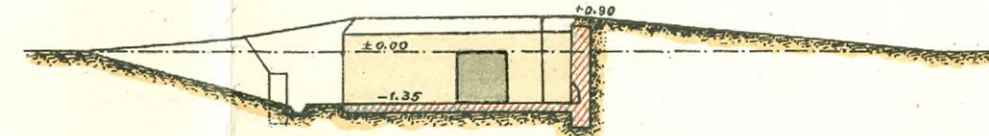
Разрѣзъ по № 6
