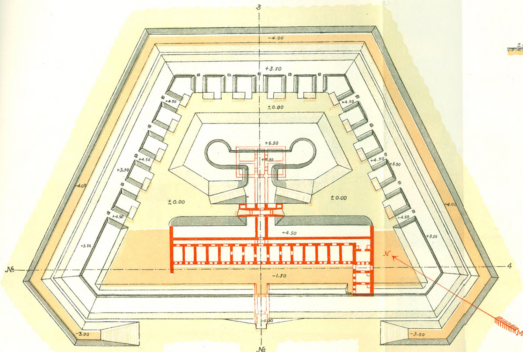
I. Фортъ Хадърлъкъ
