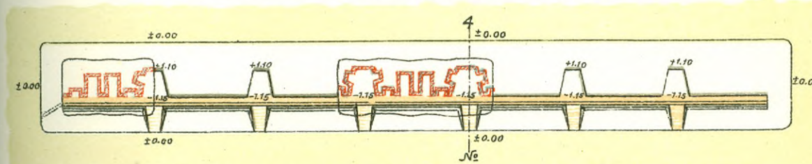
Батарея за 15 см. крепостни оръдия.
