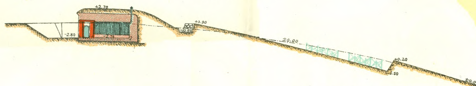
Разрѣзъ по № 6
