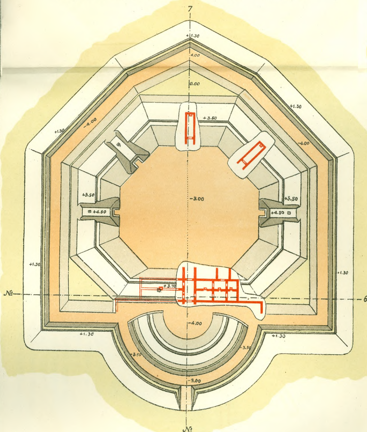
XIV. Фортъ Айжи-Йолу
