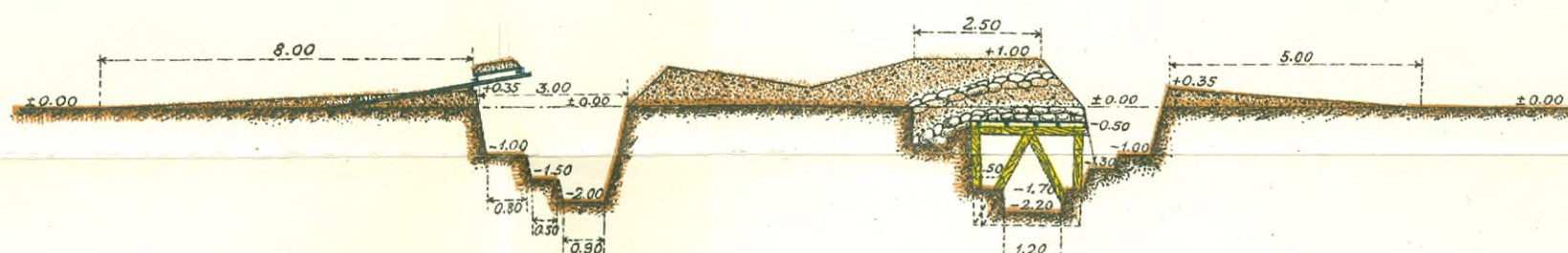
Разрѣзъ по № 2
