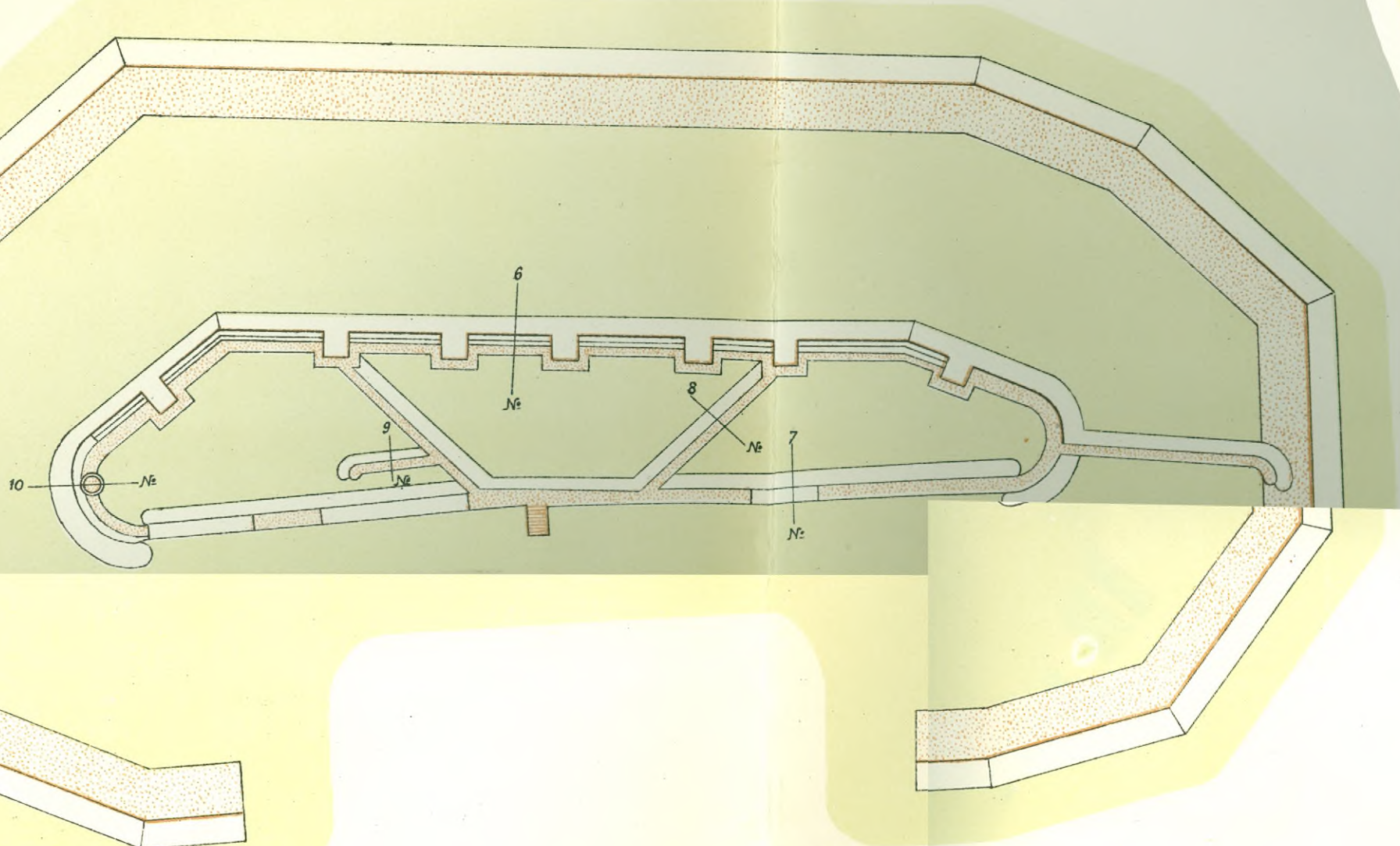
Редута при гробищата. Въ С. Западна секторъ.
