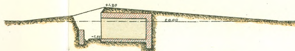
Разрѣзъ по № 7
