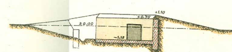
Разрѣзъ по № 4
