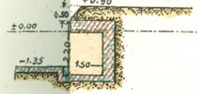
Разрѣзъ по № 8
