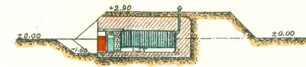
Разрѣзъ по № 10
