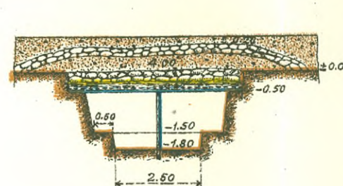
Разрѣзъ по № 2
