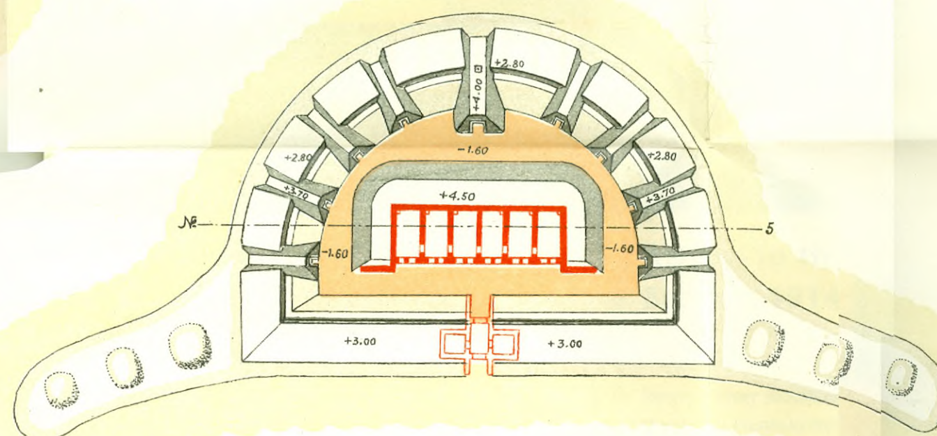
IV. Фортъ Айналъж
