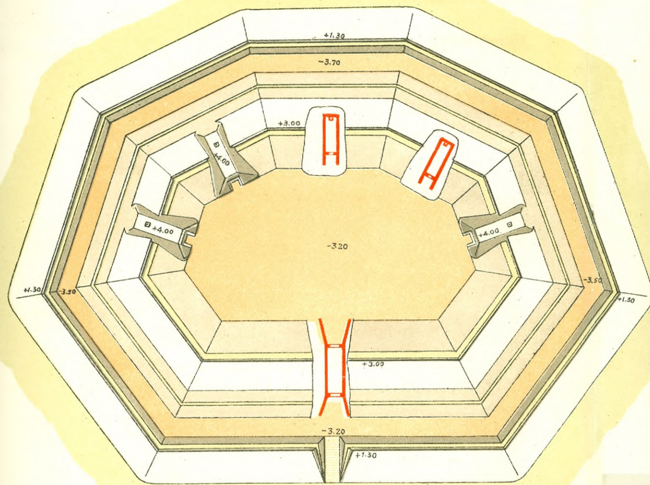
XIV. Фортъ Айжи-Йолу
