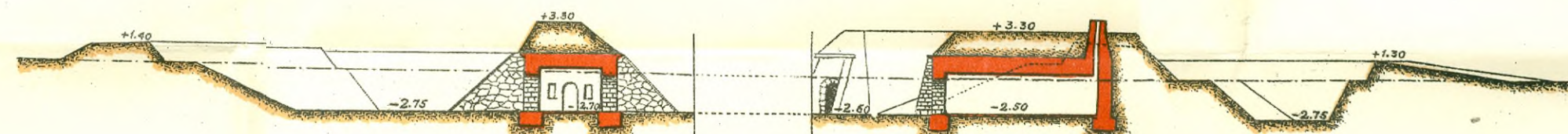
Разрѣзъ по № 5
