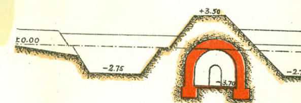
Разрѣзъ по № 1
