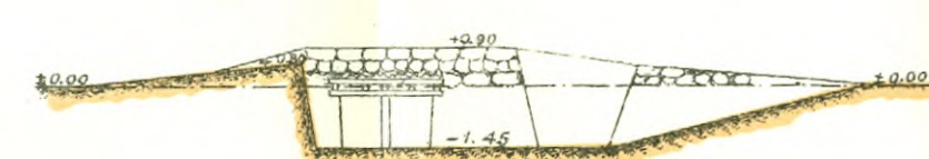
Разрѣзъ по № 1
