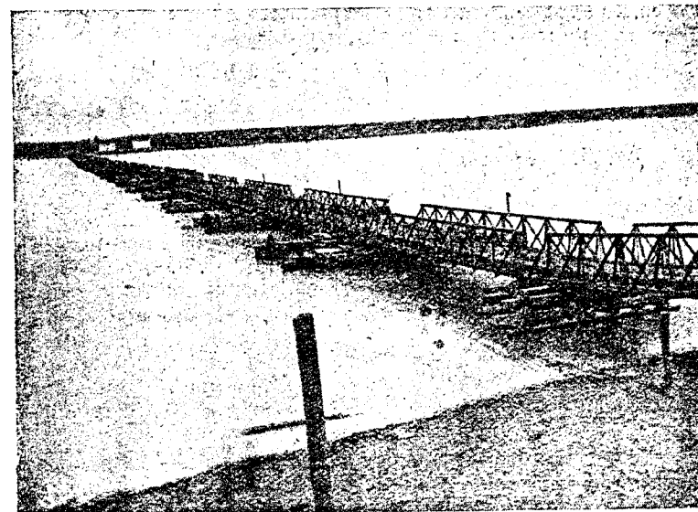
Мостътъ надъ р. Дунавъ отъ Свищовъ за Зимничъ.
